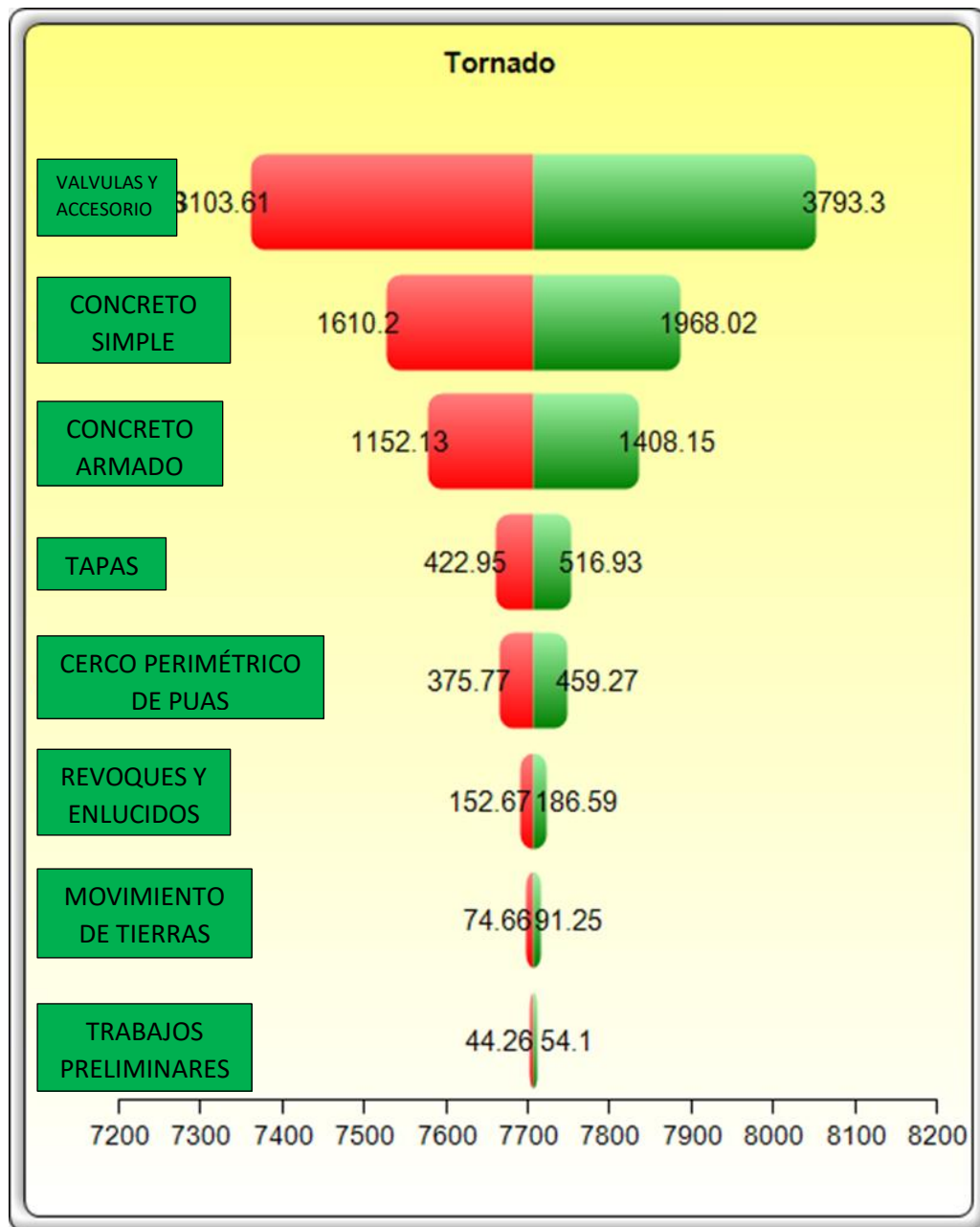
Figura 8. Análisis Tornado Título 02.01 Captación en Quebrada
